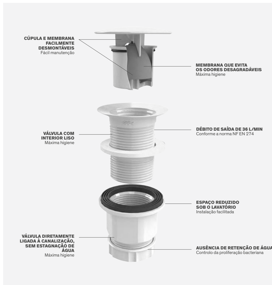
Corte 3D_621W: válvula sem água Ref. DELABIE: 621W
