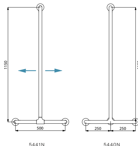
Colocação da barra vertical regulável (ref. 5441N)
