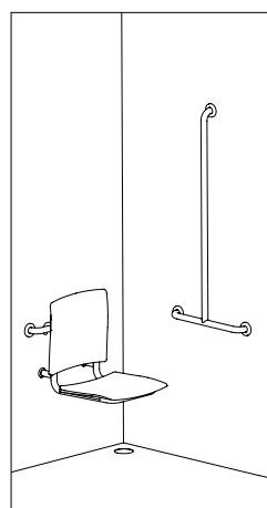
Exemplo de instalação num duche
