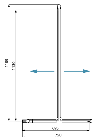
Colocação da barra regulável à esquerda ou à direita
