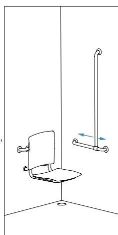
Colocação da barra vertical (ref. 5441)
