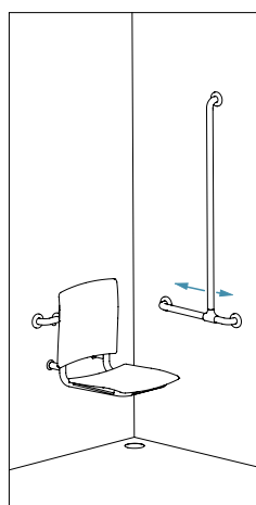
Colocação da barra vertical regulável (ref. 5441N)
