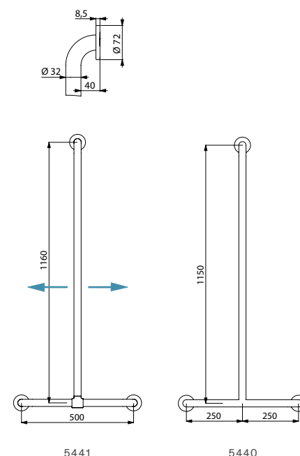
Colocação da barra vertical (ref. 5441)
