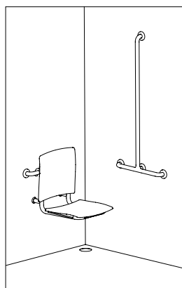
Exemplo de instalação num duche
