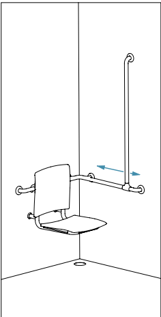
Colocação da barra vertical regulável à esquerda ou à direita (ref. 5481N)
