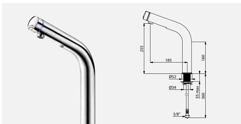
Misturadora de lavatório temporizada TEMPOMIX 3 H. 250 Ref. DELABIE : 794120
