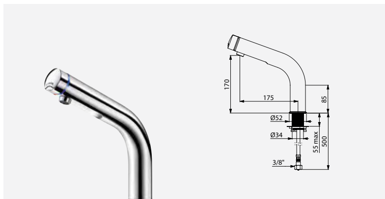
Misturadora de lavatório temporizada TEMPOMIX 3 H.170 Ref. DELABIE : 794110
