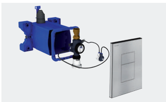
TEMPOFLUX 3 encastrar Ref. DELABIE : 763BOX-763000
