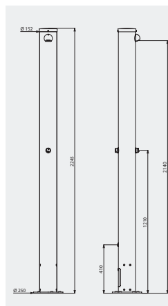
Coluna de duche AR LIVRE com 1 duche e 1 lava-pés Ref. DELABIE - 717511
